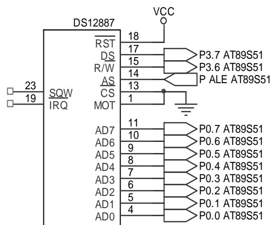
Gambar 8. Rangkaian DS12887
